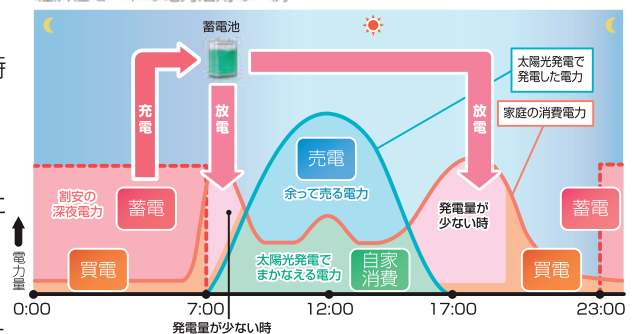
クリーンモードの電力活用の一例
